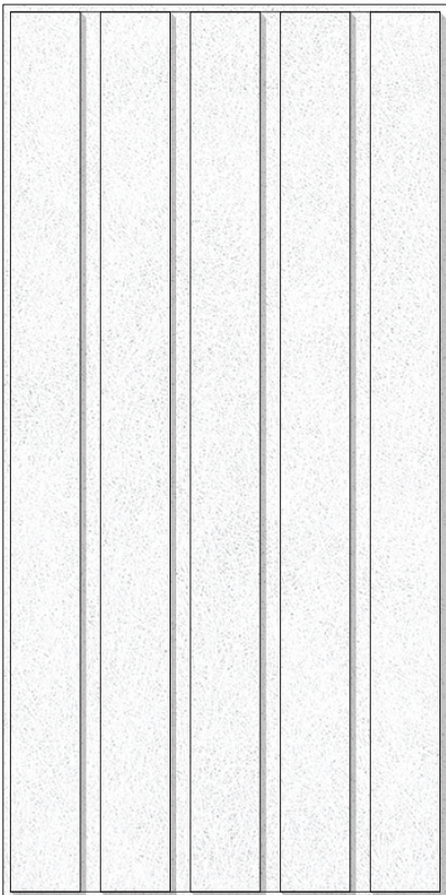
Troldekt® tiles 5, T24 25 x 593 x 1193 mm
